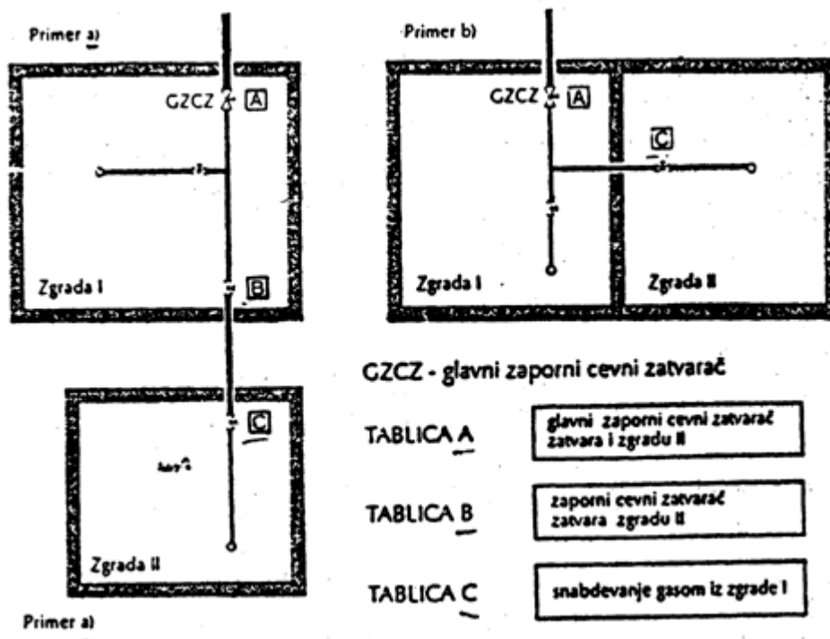
Slika 1 - Primeri ugradnje i označavanje zapornih cevni zatvarača
